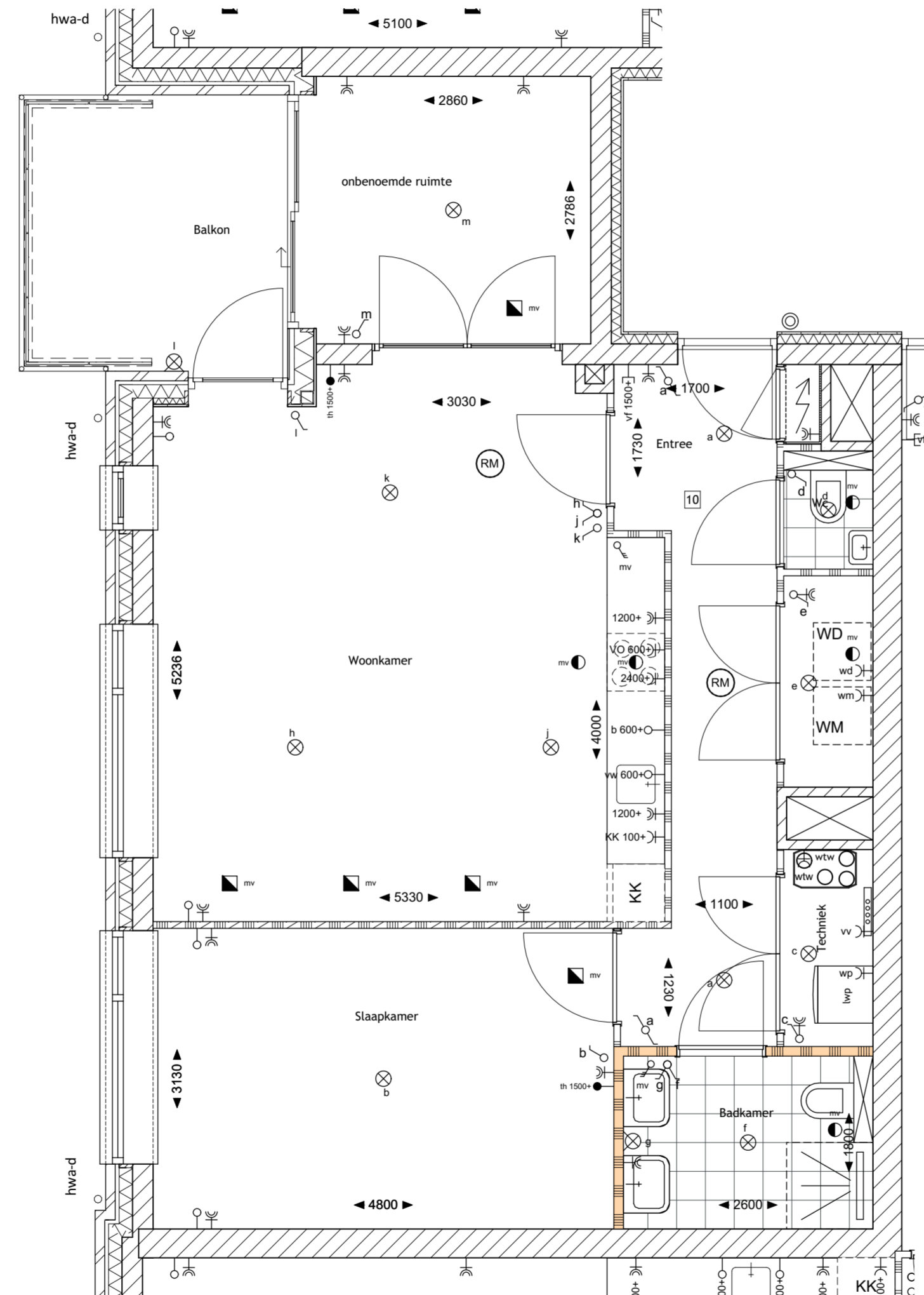
Plattegrond - Type C2 Optie dubbele deuren in woonkamer Bnr.: 10 1:50
